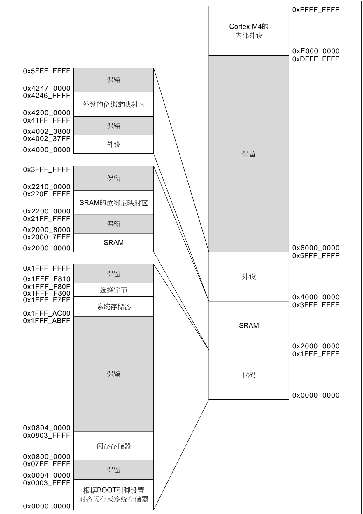
图 7. 存储器图
